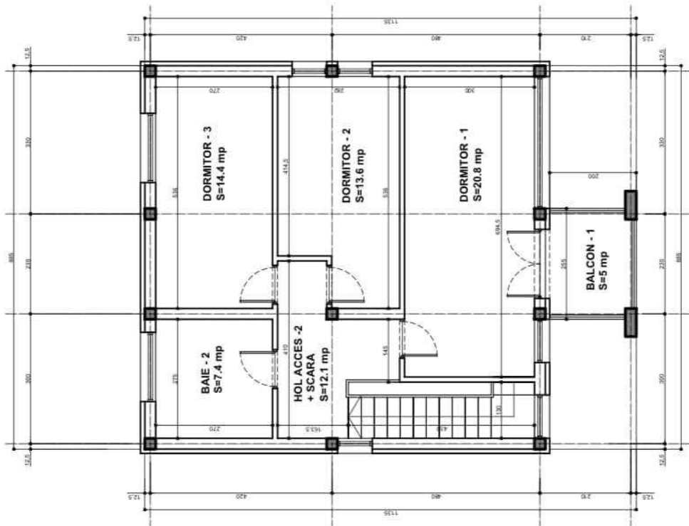
Plan etaj Scara 1:50
